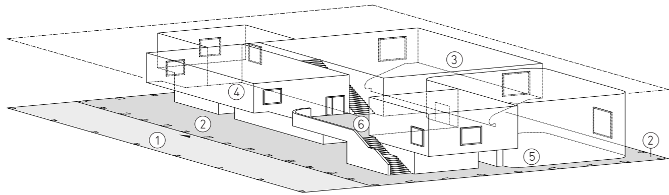
Isometrie Wandelhalle
