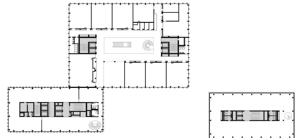
2. Obergeschoss
