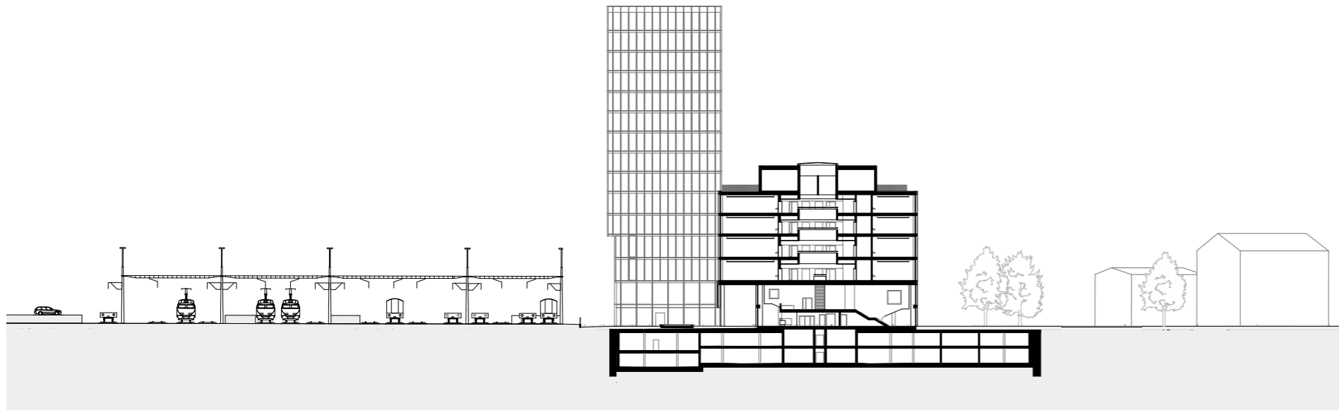
Querschnitt
